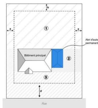
Croquis 2 : Abri d'auto permanent
