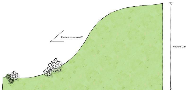
Croquis 7 : Hauteur d'un talus
